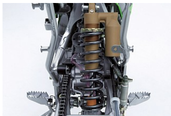
Задний амортизатор
