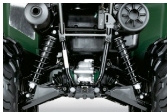
Задняя подвеска
