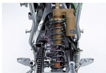
Задний амортизатор
